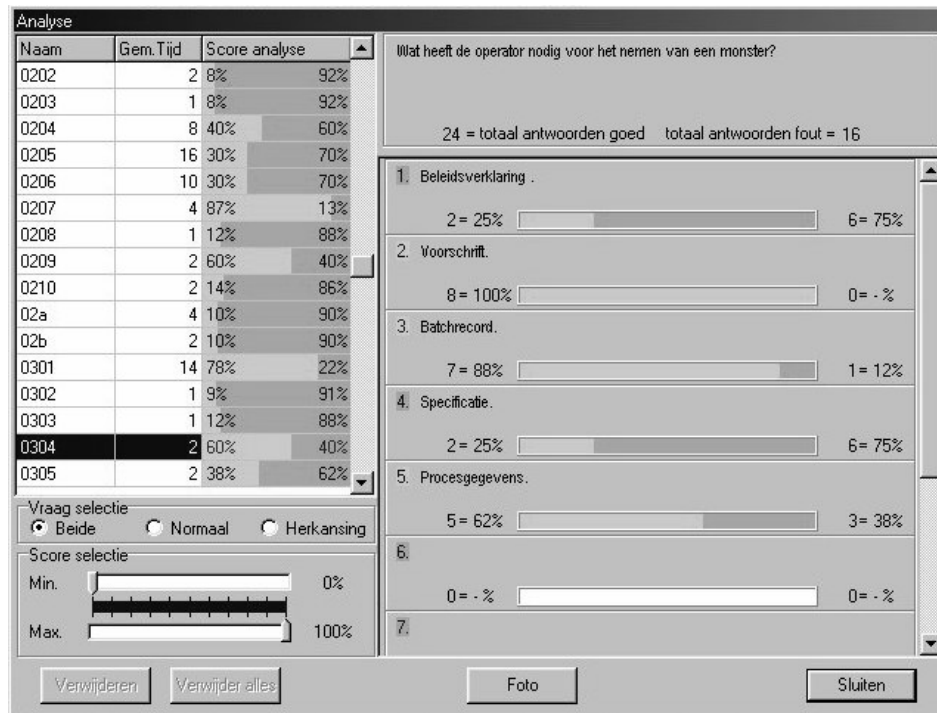
Figuur 4.6: Analysescherm Registratiesysteem GMP +
