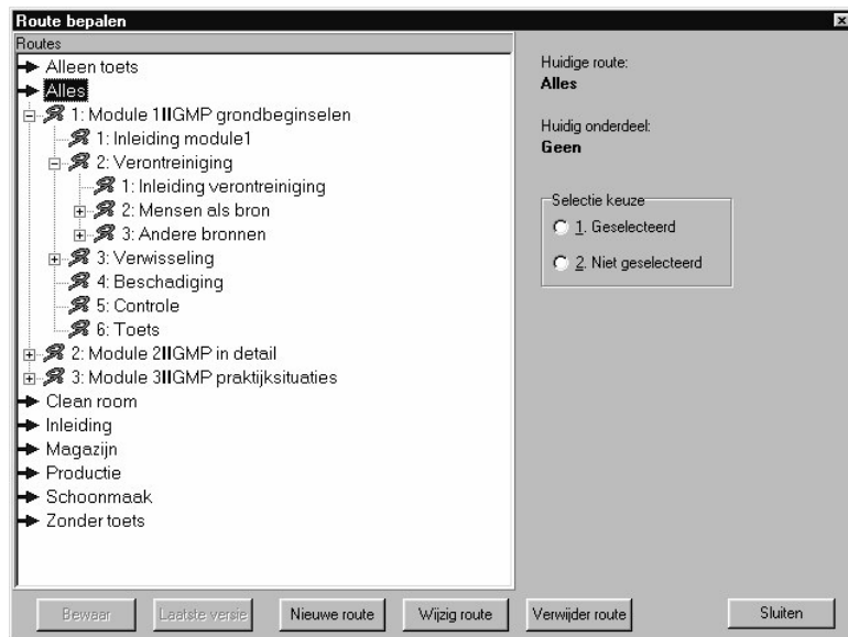
Figuur 4.7: Routescherm van het Registratiesysteem GMP 1
